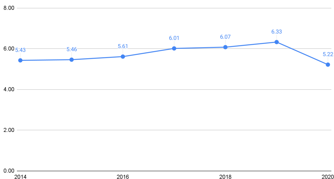
Figura 59: Emisiones de toneladas de CO 2 e por persona (2013-2020) (Basic). Fuente: Elaboración propia
