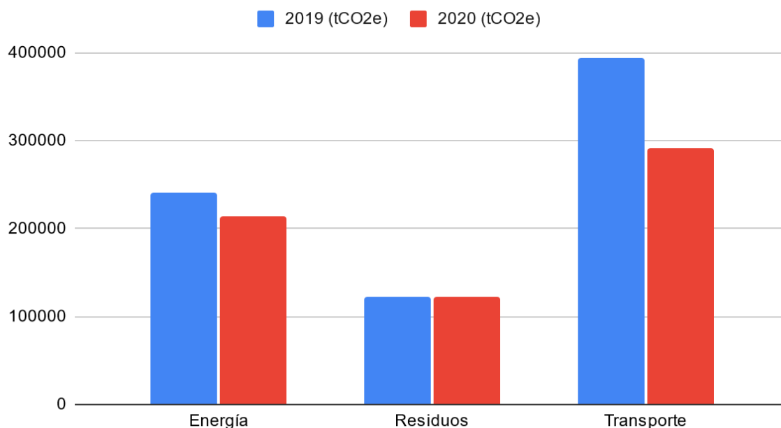
Figura 58: Análisis comparativo por factor entre los IGEI del año 2019 y 2020 del Municipio de Ciudad de Mendoza (Basic).
