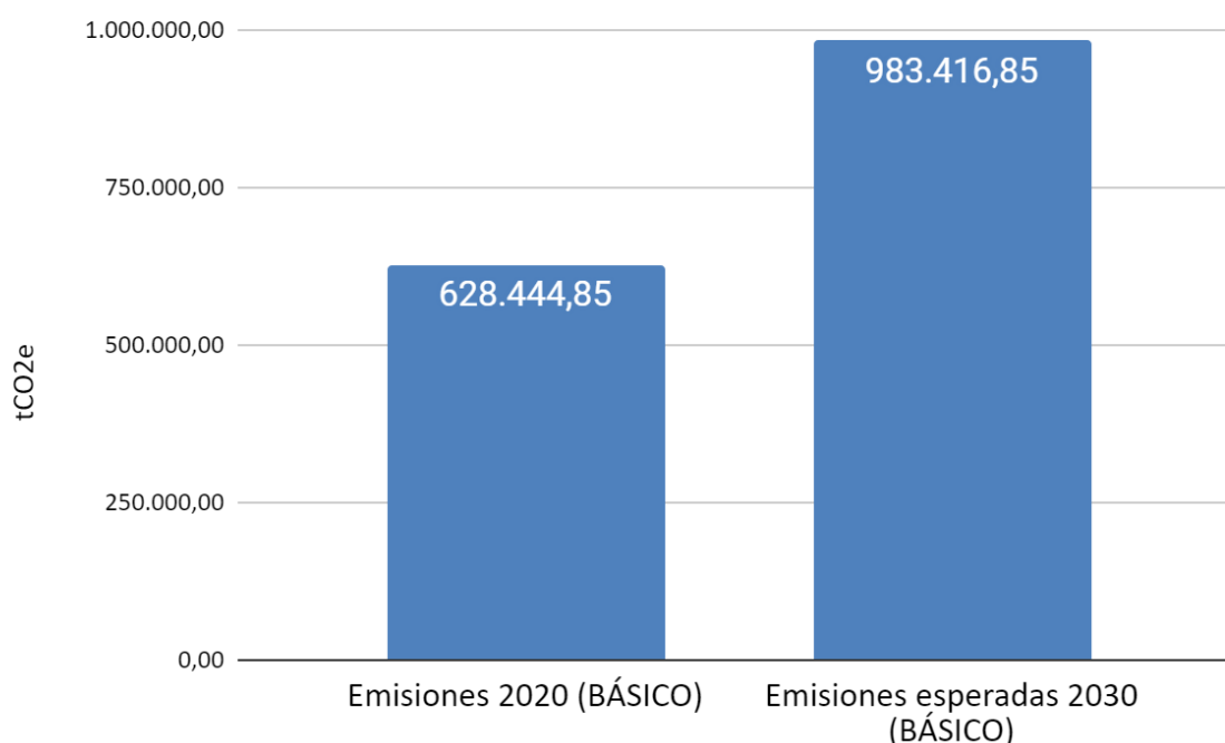
Figura 75: Escenario de referencia BAU. Fuente: RAMCC 2023.
